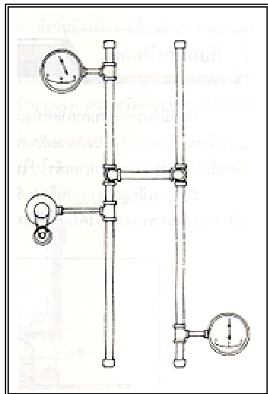
รูปที่ 8 การต่อท่อแบบวงจรถัดทำให้การไหลของอากาศไม่สะดวกและระดับสูญญากาศไม่คงที่
